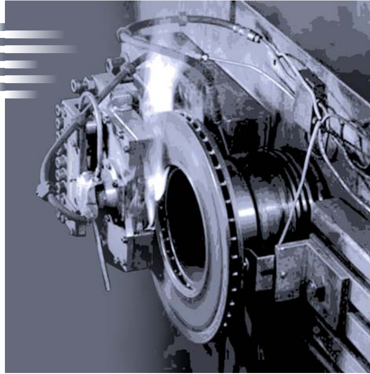
Telemetriesender montiert auf Prüfstandswelle (geteilter Senderträger für Klemmontage)
