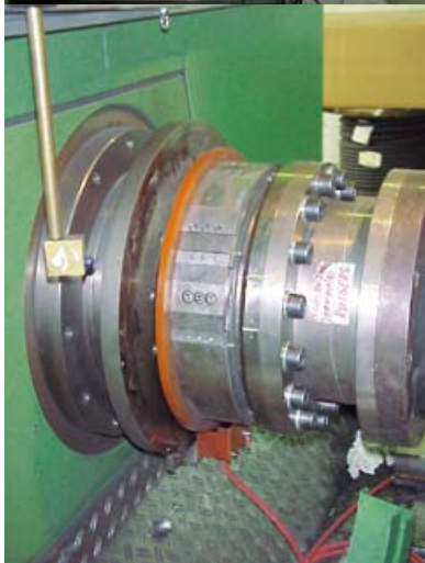
Telemetriesystem integriert in den Prüfstandsflansch (Schenck Pegasus LKW-Bremsenprüfstand)
