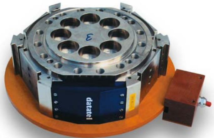
Telemetriesystem integriert in den Prüfstandsflansch (Schenck Pegasus PKW-Bremsenprüfstand)
